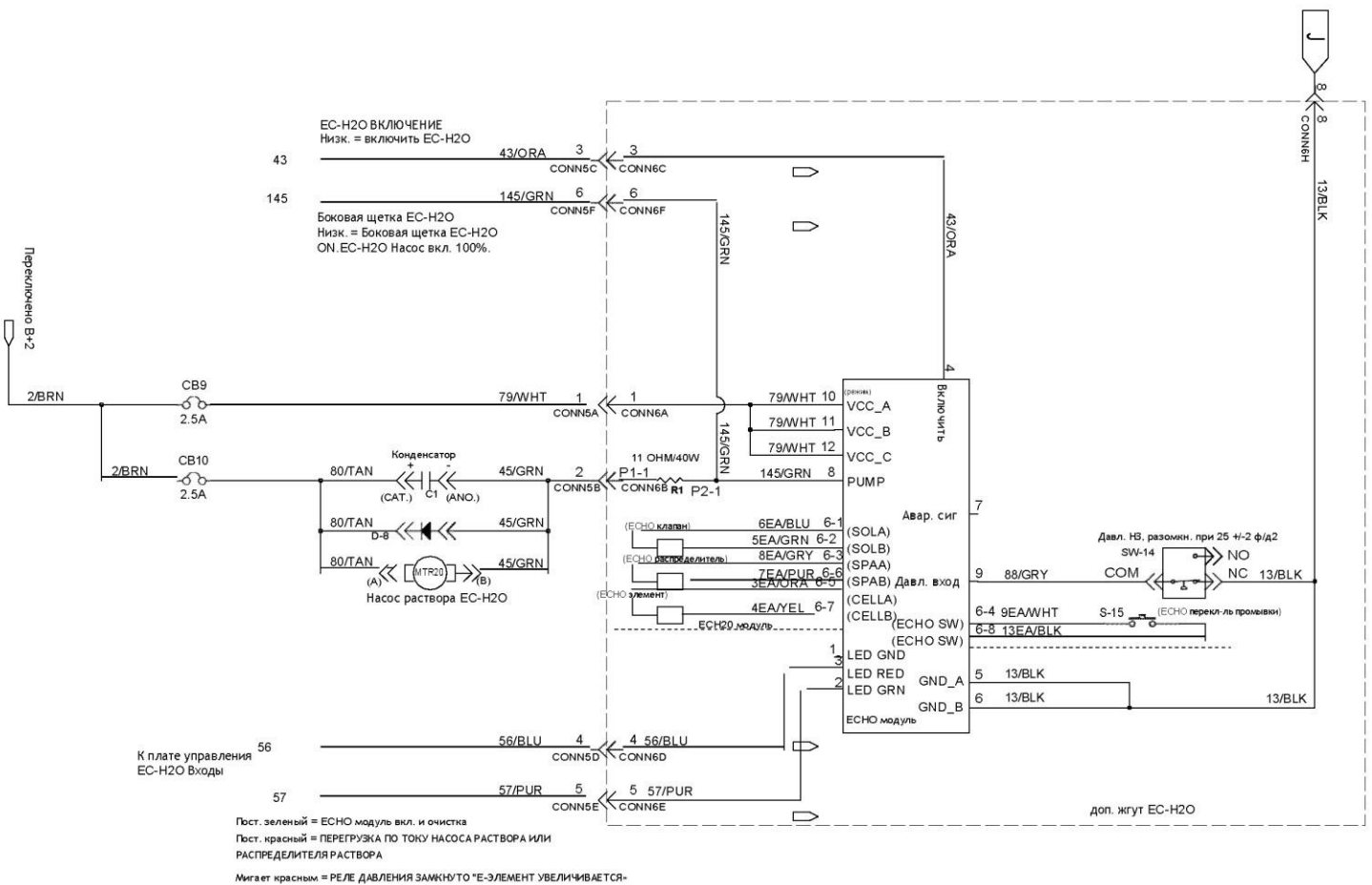
Схема электрическая принципиальная (6 из 6)
